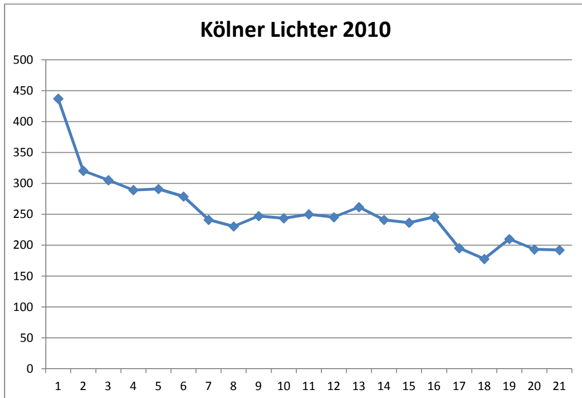
Abb. 4.: Personenstrom beim Veranstaltungsende der Kölner Lichter. (Anzahl der Personen pro Minute gegen die Zeit in Minuten)
