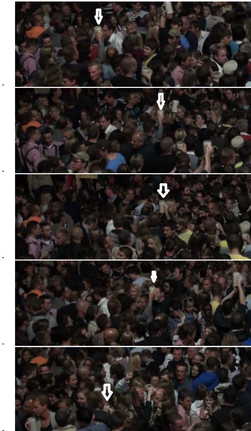
Bild 13: Erzwungene Bewegung eines Besuchers durch Gegenstrom
